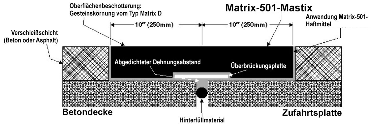
Abbildung 1. Typischer Einbau des BB-Joint-M-501 Asphaltic Plug Bridge Joint System.
